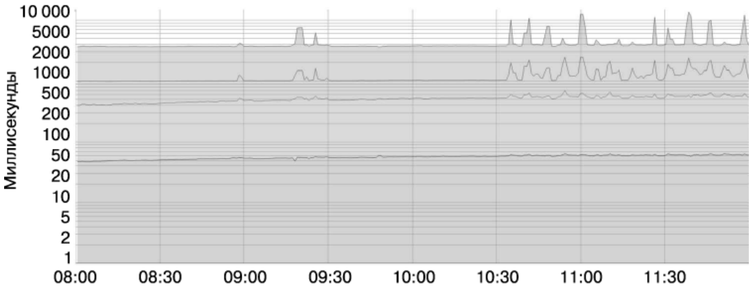
Рис. 4.1. Показаны 50-й, 85-й, 95-й и 99-й перцентили задержки системы. Обратите внимание на то, что ось Y имеет логарифмическую шкалу
