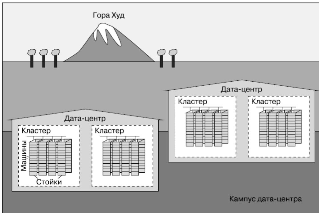
Рис. 2.1. Пример топологии кампуса дата-центров Google
