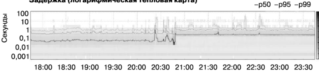
Рис. 12.4. Задержка приложения. Кривые на графике соответствуют величинам задержки, в которые укладывается выполнение соответственно 50, 95 и 99 % запросов. «Карта нагрева» показывает, сколько запросов попадает в каждый интервал
